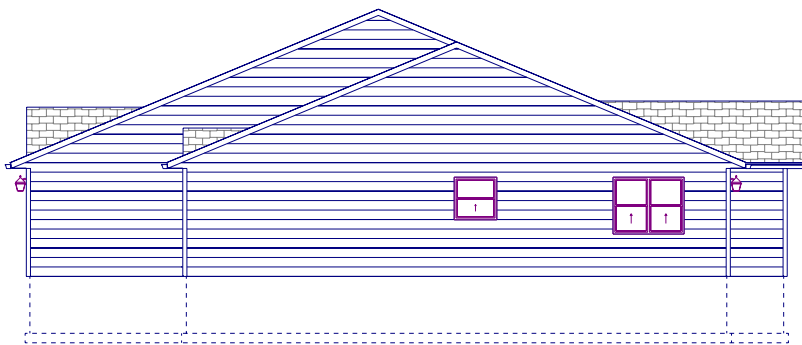
RIGHT ELEVATION
